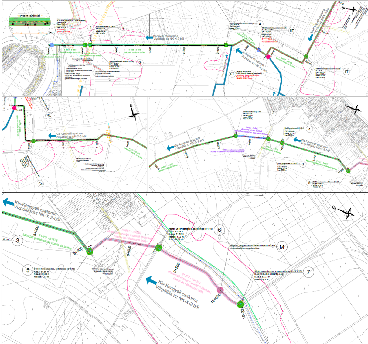
7. ábra: Részletes helyszínrajzok (forrás: VIZITERV Environ Kft.)
