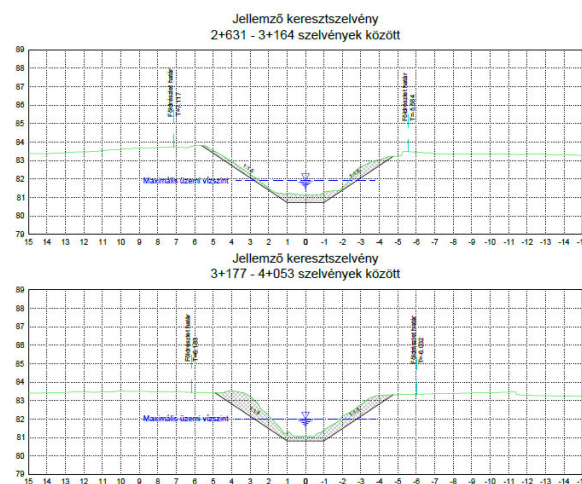
6. ábra: Kengyeli-főcsatorna – Kis-Kengyeli-csatorna jellemző keresztszelvényei (forrás: VIZITERV Environ Kft.)
