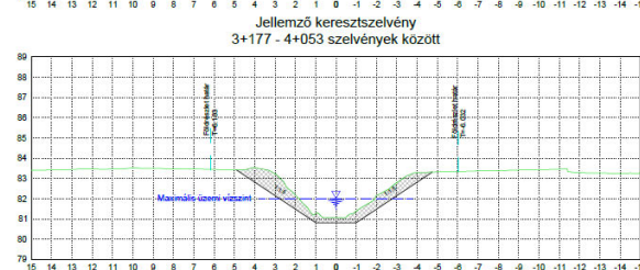
6. ábra: Kengyeli-főcsatorna – Kis-Kengyeli-csatorna jellemző keresztszelvényei (forrás: VIZITERV Environ Kft.)
